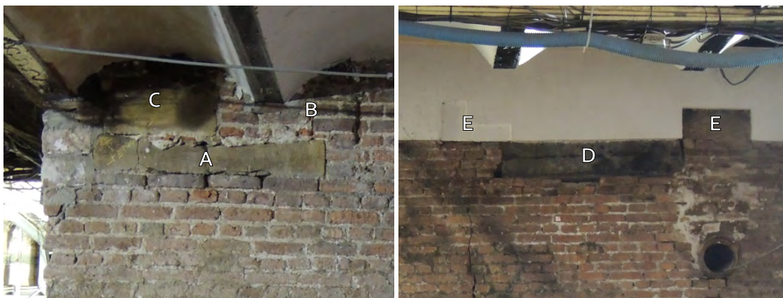
40 Dichtgezette doorgangen met zandstenen (links) en hardstenen (rechts) onderdorpel
